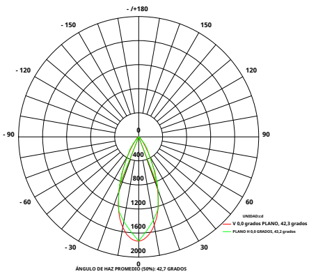
Proyector (40°)
